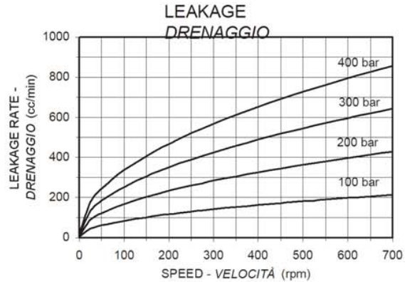
LEAKAGE RATE DRENAGGIO
