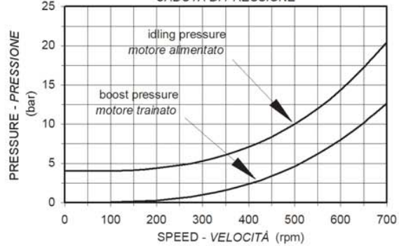
IDLING AND BOOST PRESSURE CADUTA DI PRESSIONE
